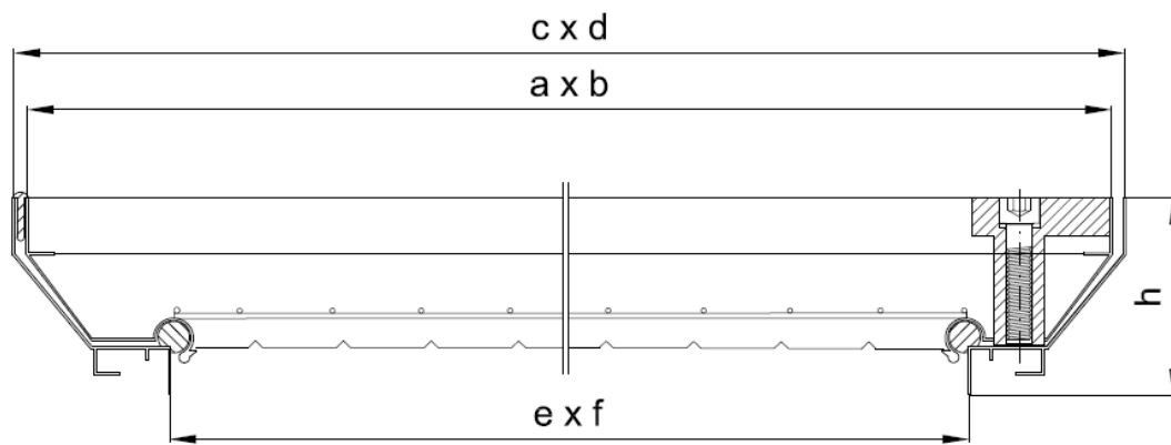
e x f - całkowity prześwit włazu a x b - zewnętrzny wymiar pokrywy c x d - zewnętrzny wymiar ramy h - wysokość ramy
